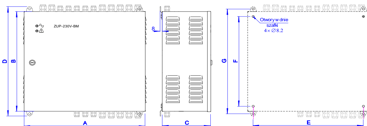
Rys.1.b. Gabaryty i rozstaw otworów mocujących zasilaczy ZUP-230V-BM w szafce typu M i L .
