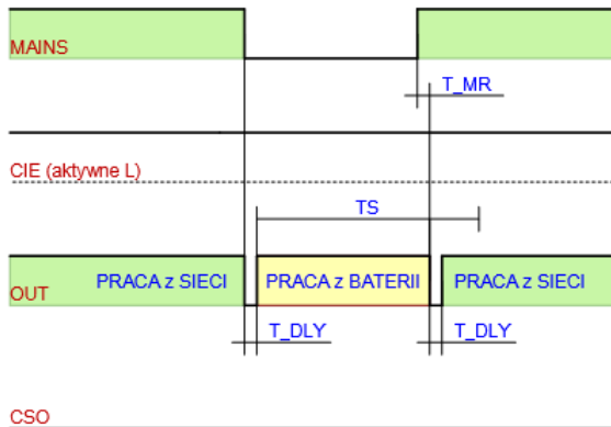
Rys. 10a. (poniżej) Powrót zasilania sieciowego 230V podczas pracy bateryjnej wywołanej alarmem pożarowym, z przerwaniem pracy bateryjnej.
